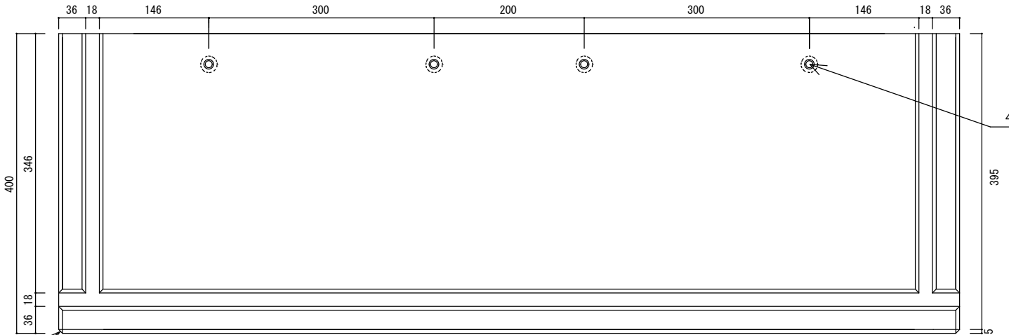
【底面図】
