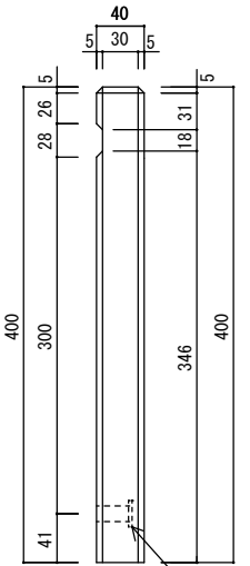
【側面図】 4-W3/8×30インサート
