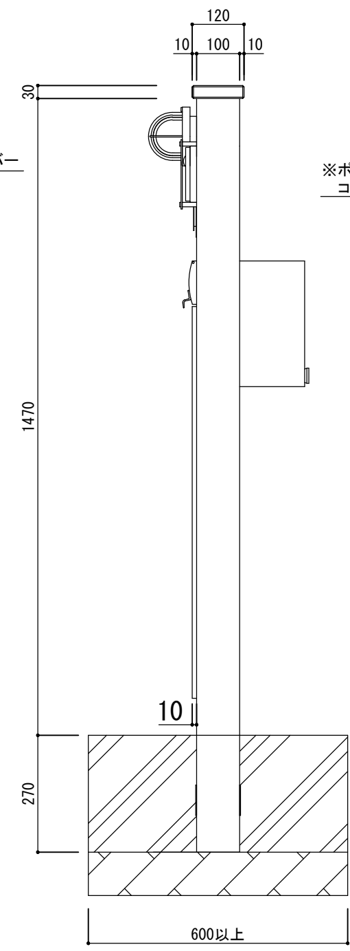
【右側面図】
