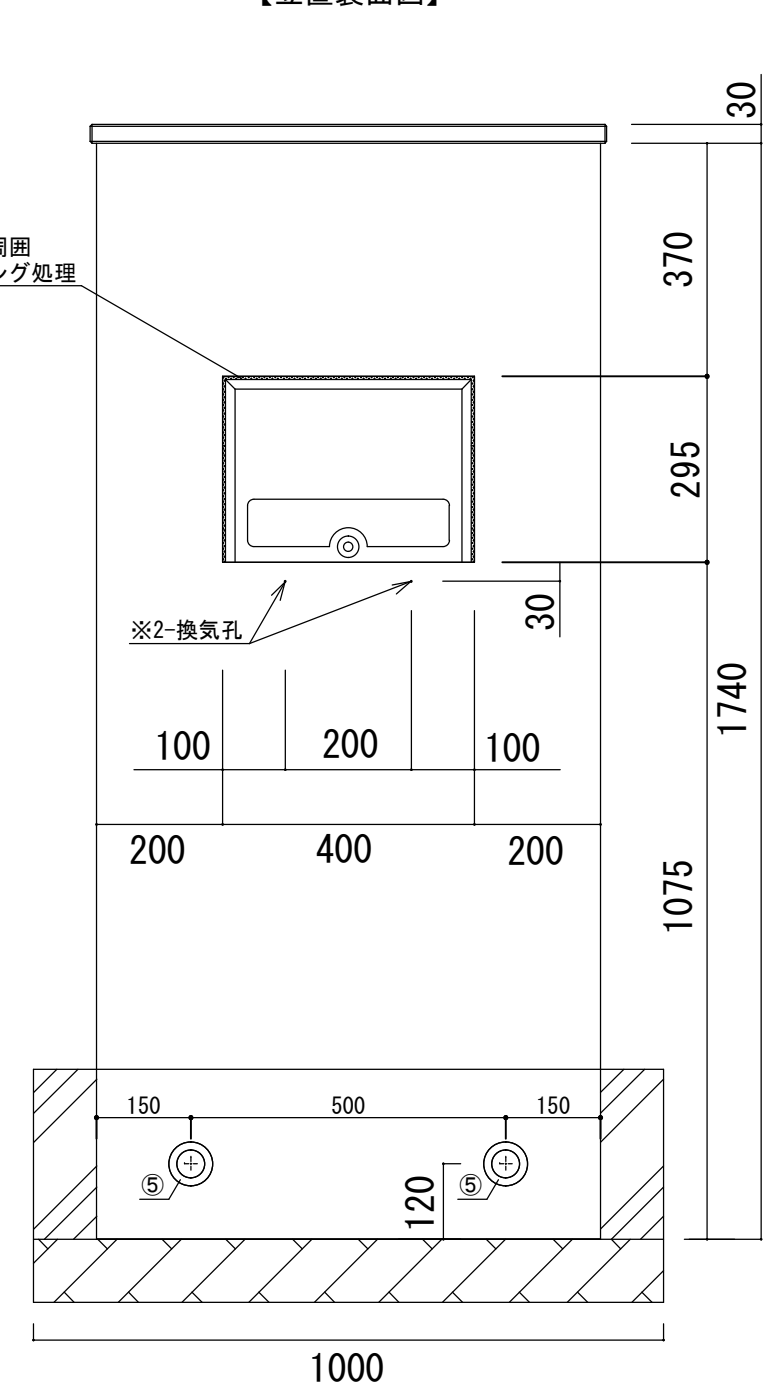
【笠置裏面図】
