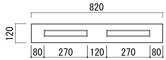
【笠置裏面図】
