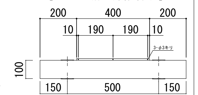
【底面図】
